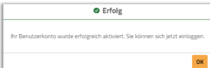
Abbildung 4-3: Erfolgreiche Aktivierung
