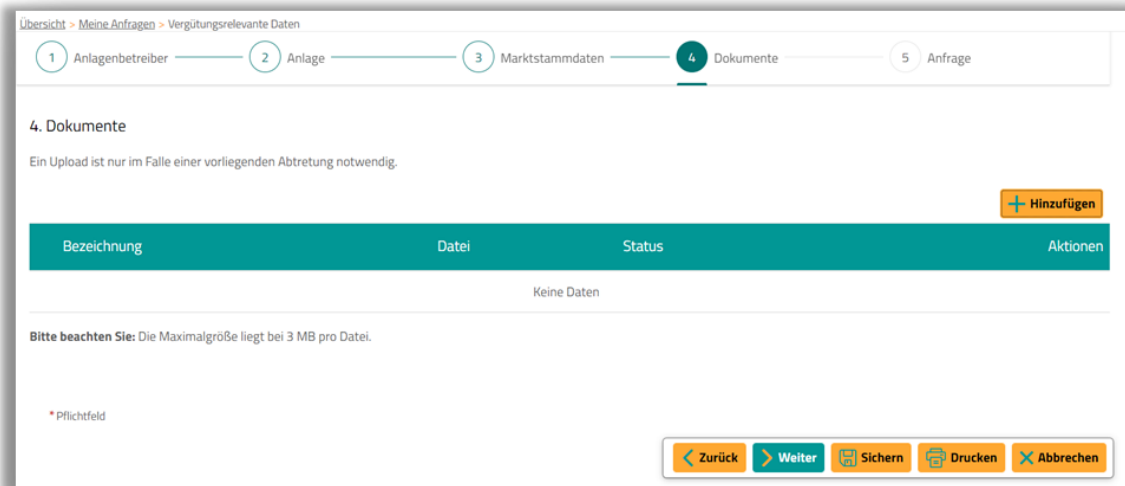
Abbildung 6-13: Maske Dokumente
